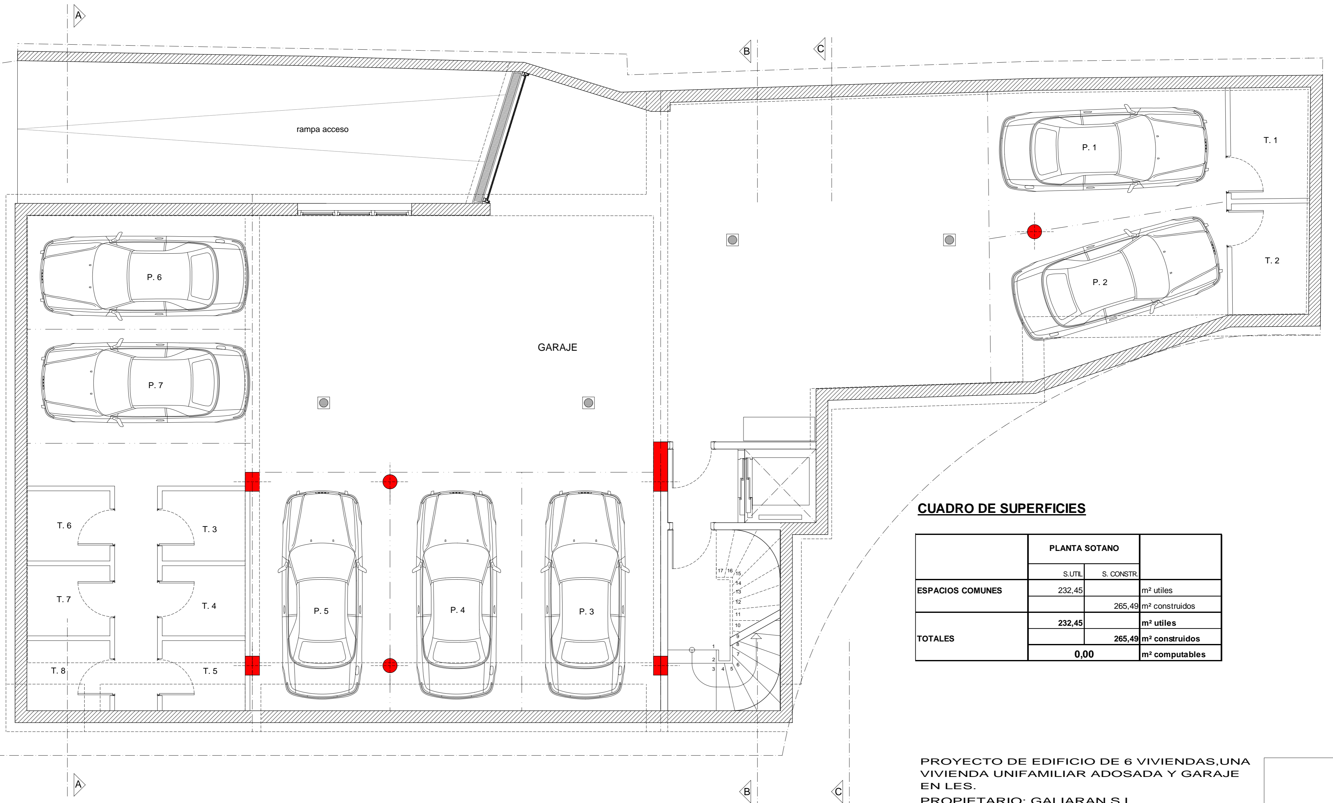
PLANTA SOTANO
