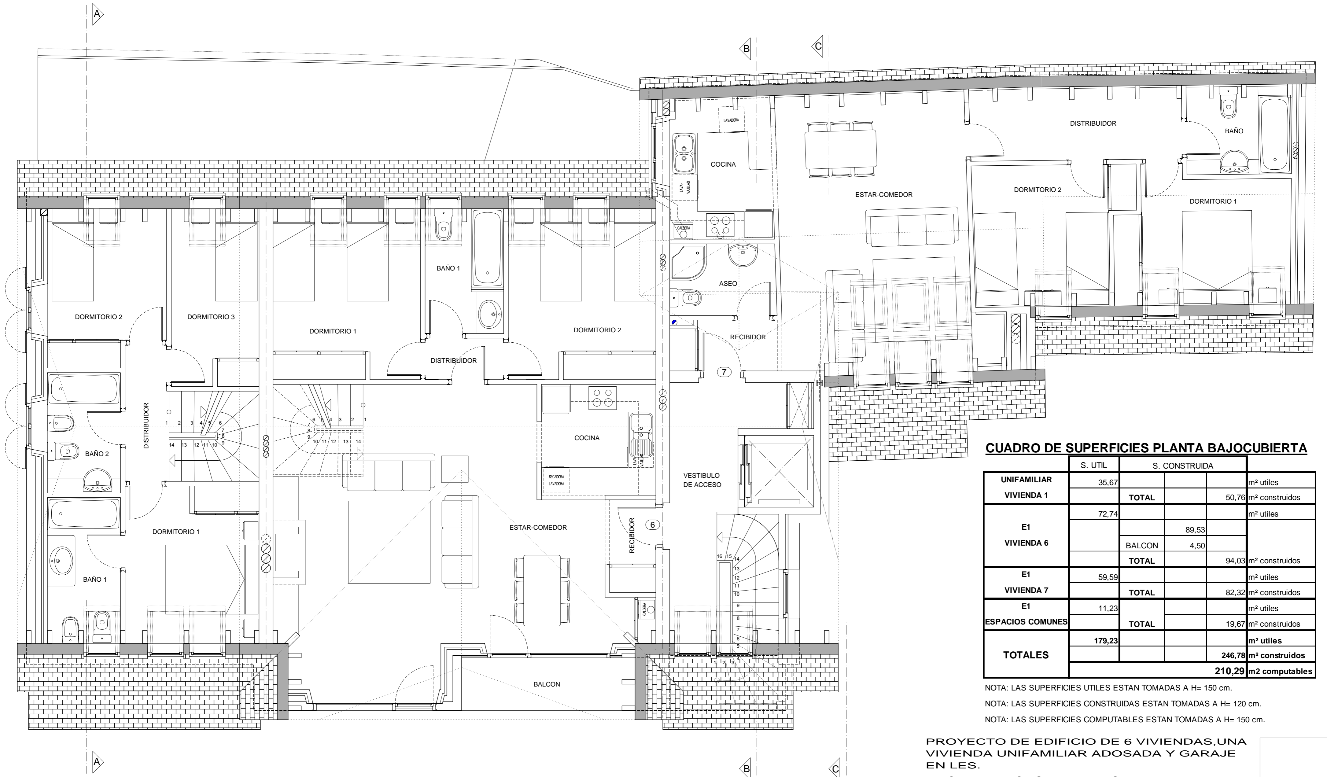
PLANTA BAJOCUBIERTA
